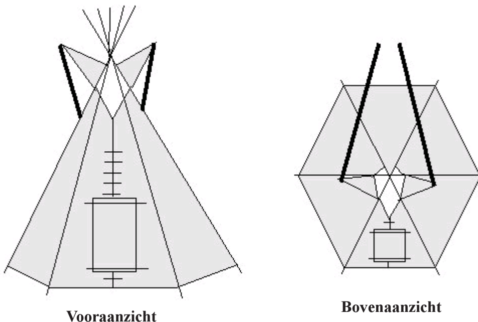
Figuur 27: Tipi met open flappen
