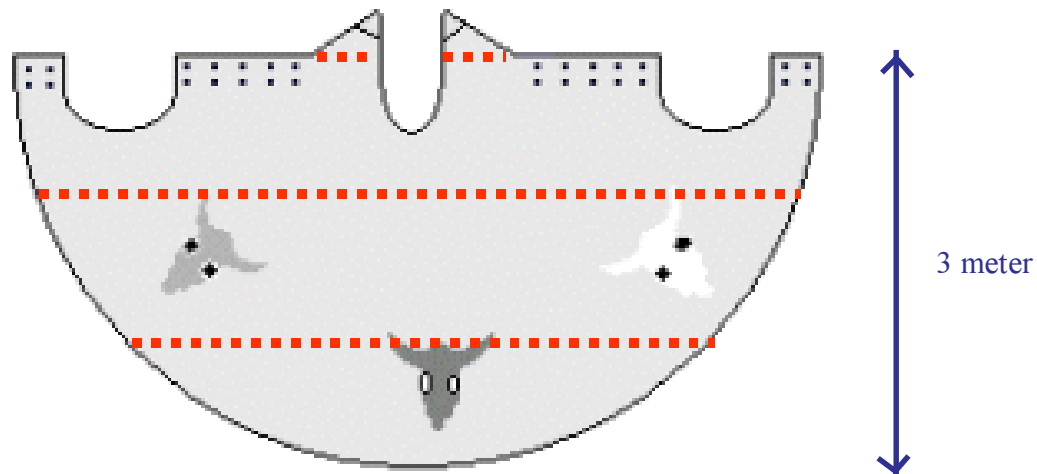
Figuur 2: Buitenzeil opgebouwd uit 3 repen katoen.
