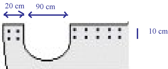
Figuur 3: Uiteinde van een buitenzeil met gaten
